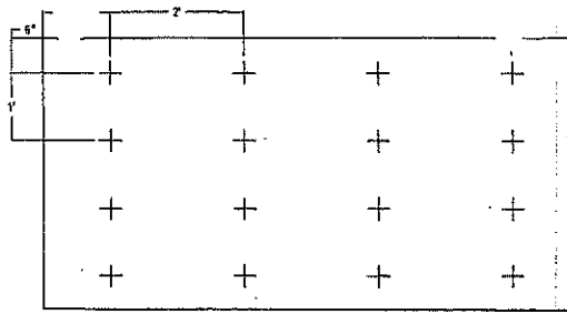
16 ANCLAJES / PLANCHA PLANTILLA PARA CENTRO: 4' X 8'
