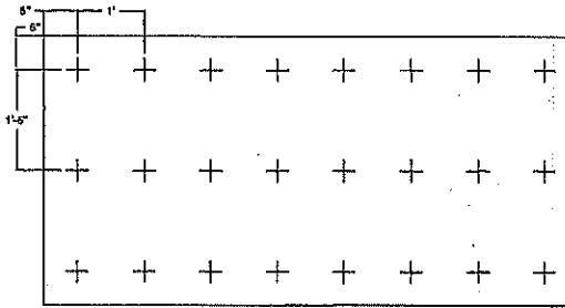
24 ANCLAJES / PLANCHA PLANTILLA PARA PERIMETRO: 4' X 8'
