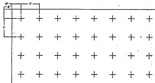
32 ANCLAJES / PLANCHA PLANTILLA PARA ESQUINAS: 4' X 8'
